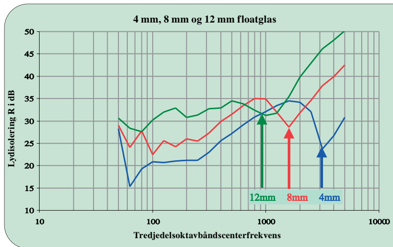
Figur 6: Glastykkelsens indflydelse på koincidensfrekvensen
