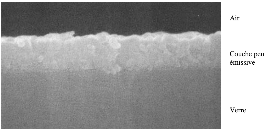
Fig.2. Coupe transversale qui montre l'uniformité du revêtement.
